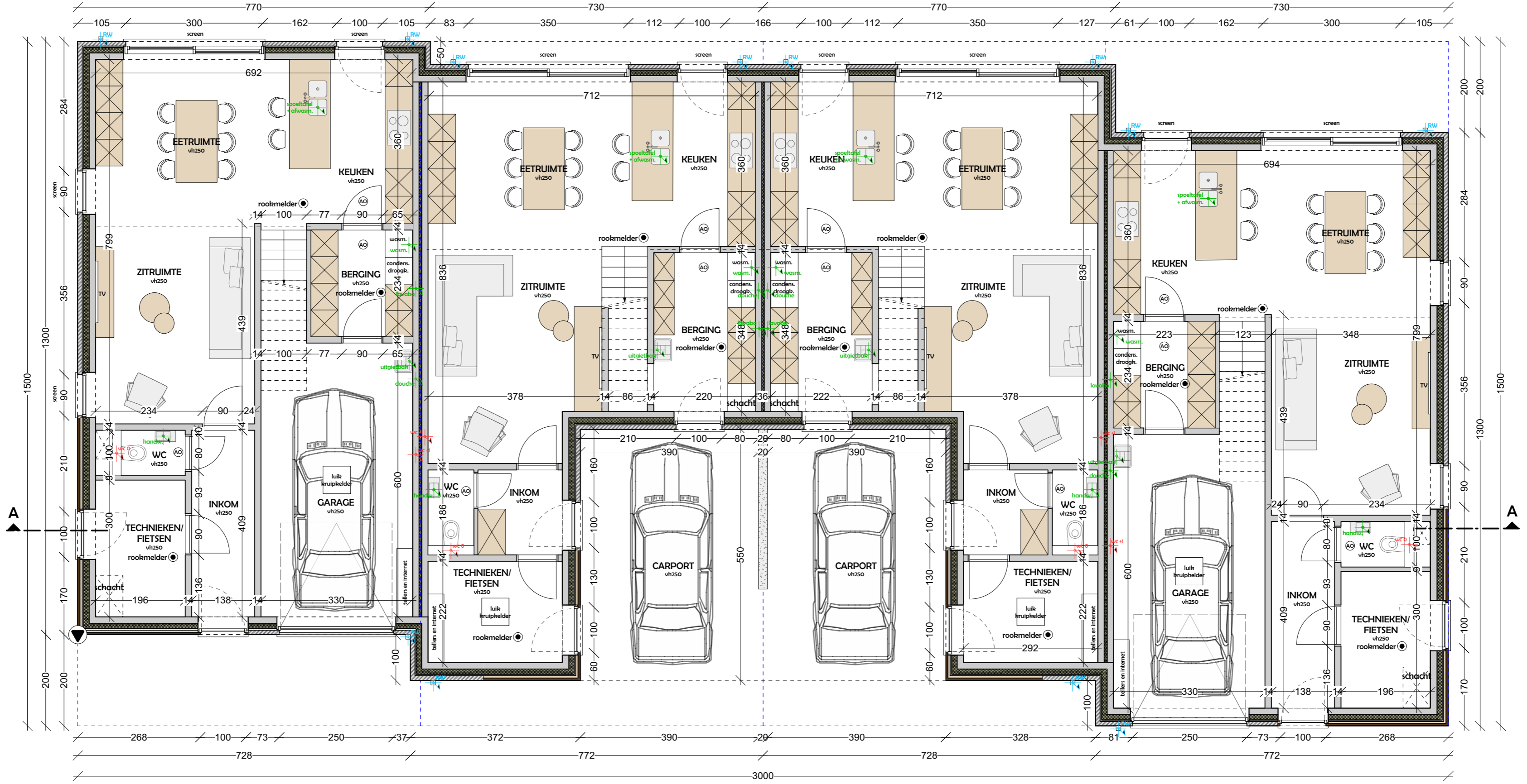
⊕ GELIJKVLOERS (loten 43 tem 46)
