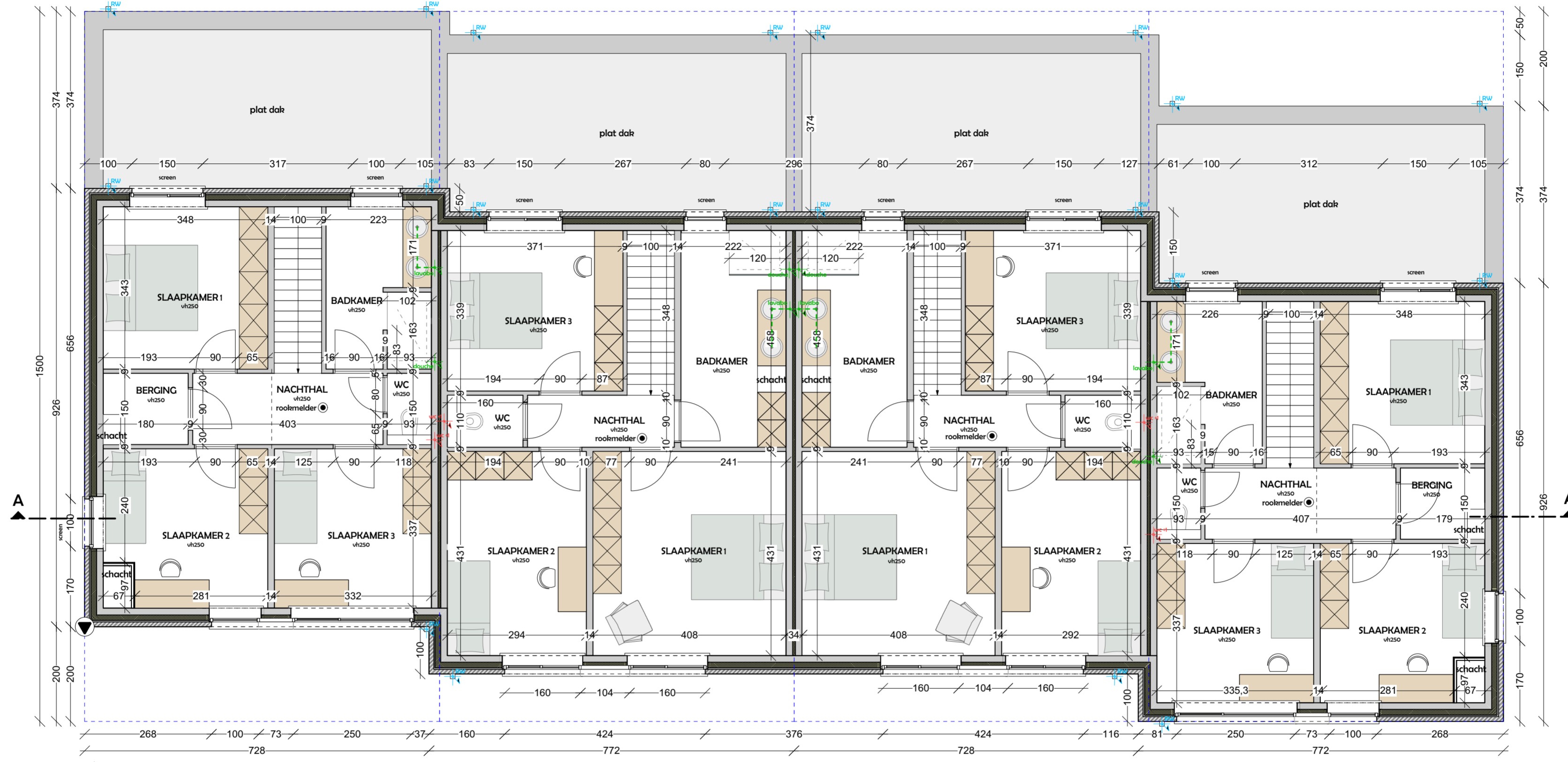
VERDIEPING (loten 43 tem 46)
